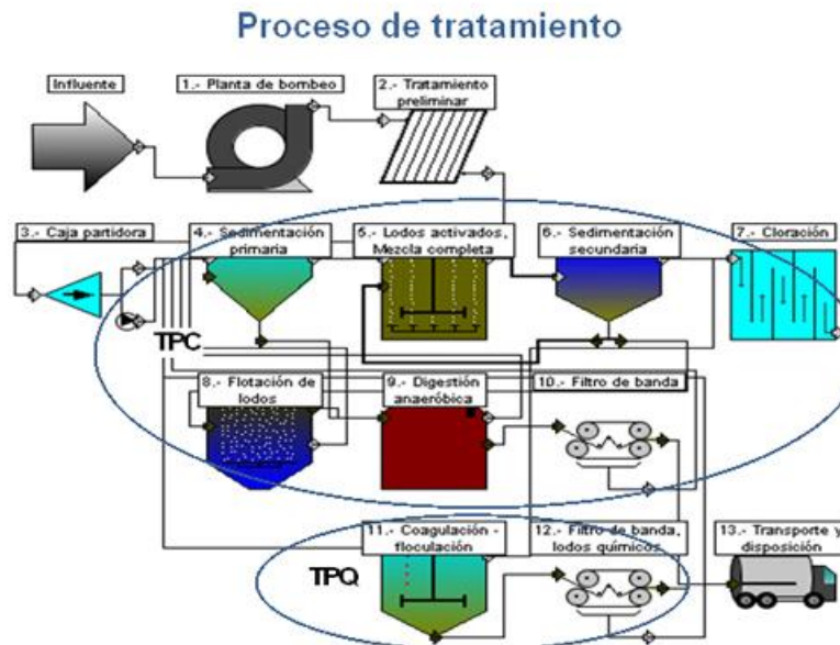
Figura 2. Planta tratadora de aguas residuales
