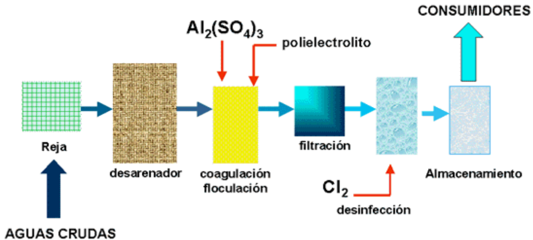
Figura 1. Tratamiento de aguas naturales
